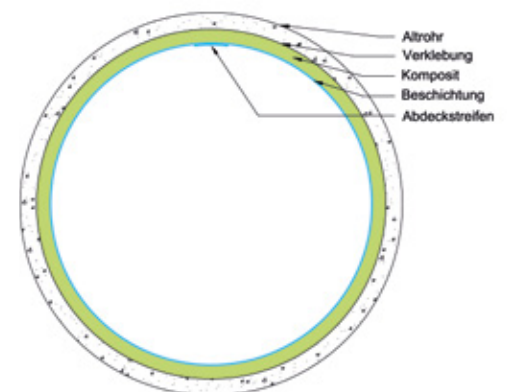
Der NORDIWALL Flex Lite dichtet Muffen und Risse ab und bewirkt eine strukturelle Verbesserung des Rohres
