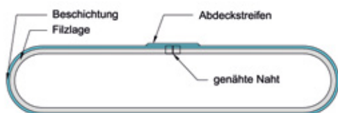
Der NORDIWALL Flex Lite ist ein beschichteter Nadelfilzschlauch
